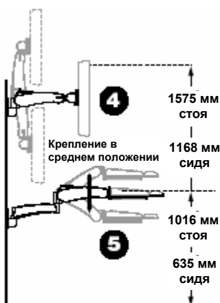
Серия 300, конфигурация для работы в положении сидя или стоя
