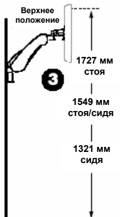
Крепление HD45
