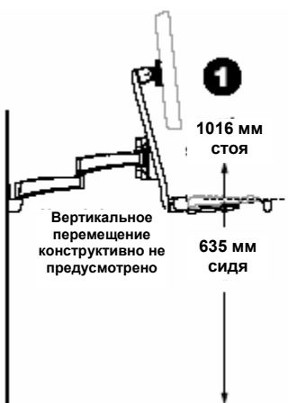
Серия 400, комбинированное крепление, конфигурация для работы в положении сидя или стоя
