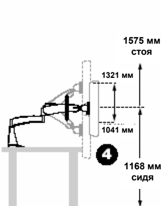
Серия 300, конфигурация для работы в положении сидя или стоя
