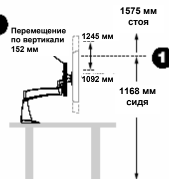
Серия 200, с вертикальным перемещением 152 мм, конфигурация для работы в положении сидя или стоя
