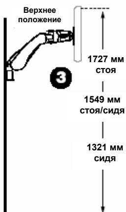
Серия HD, крепление для двух мониторов
